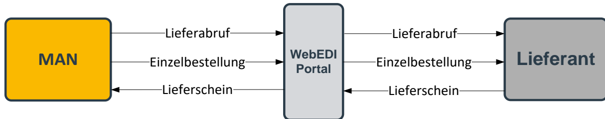
Abbildung 11 Übersicht Datenaustausch im MAN WebEDI-Portal
