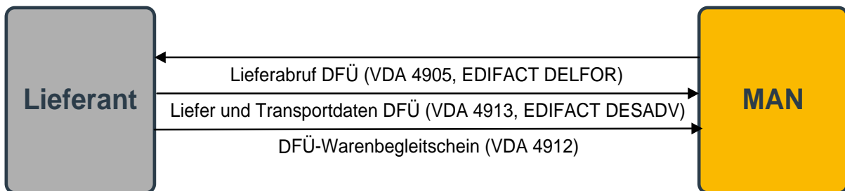
Abbildung 6 Nachrichtenaustausch Materialmanagement
